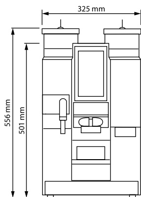
Frontansicht Maschine
