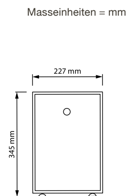
Frontansicht Milchkühler
